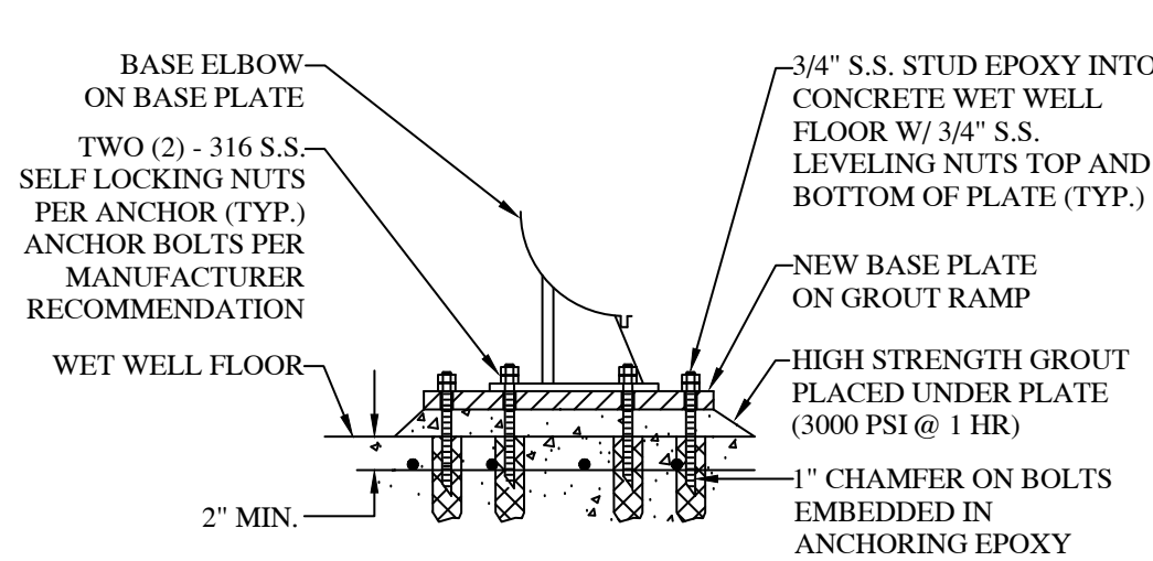
PUMP BASEPLATE SECTION DETAIL N.T.S.
